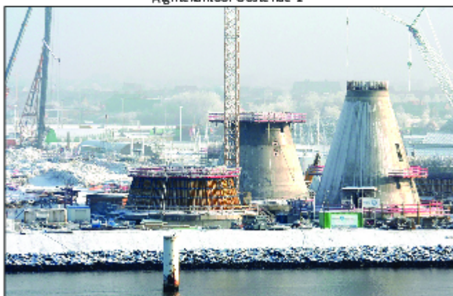
Bouw van de eerste windmolens door C-Power op de oosteroever Oostende (foto Dirk Reunbraeck, 2007)
