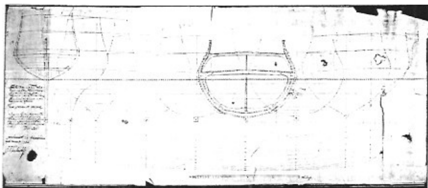
Spanttekening van de „Slesvig” (Kopenhagen, 1726) (Rigsarkivet København, Soetatens KTS, A 874)
